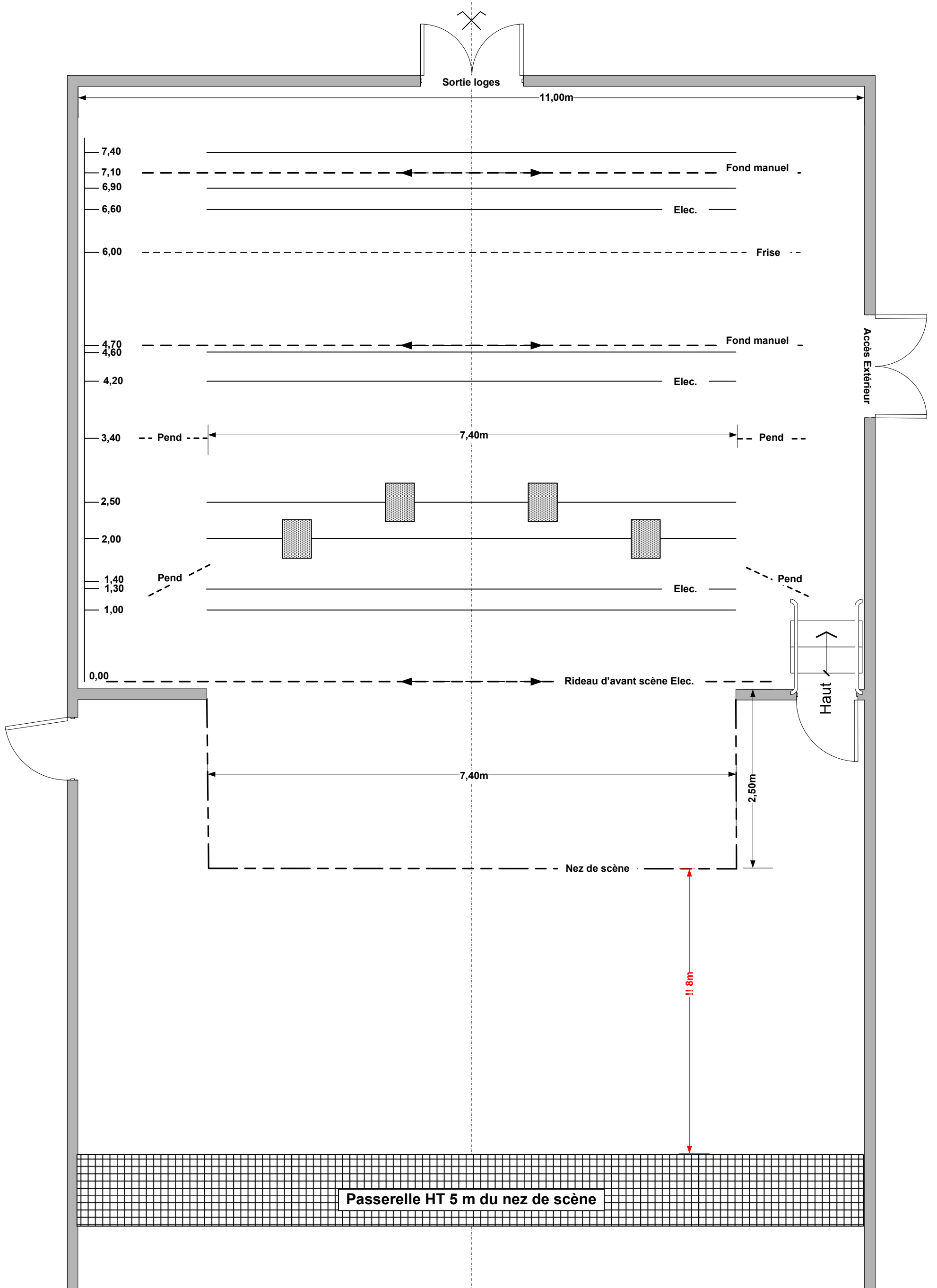
Salle de l'Alhambra – ville de Vittel Ech. 1/50
